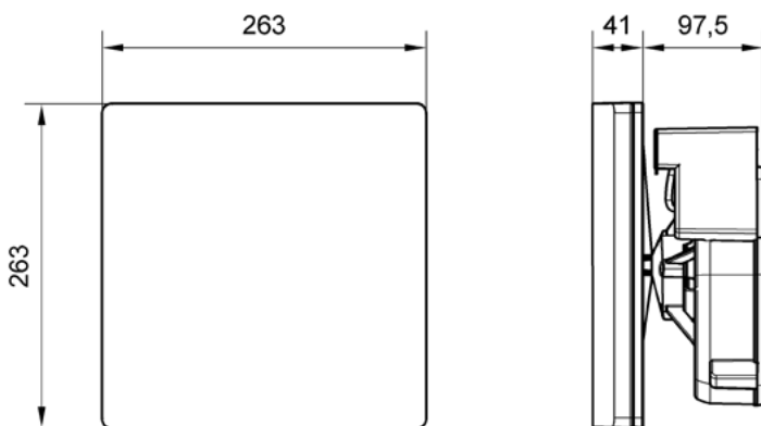
Obr. 2: Rozměry větrací vložky VARIO II v mm
